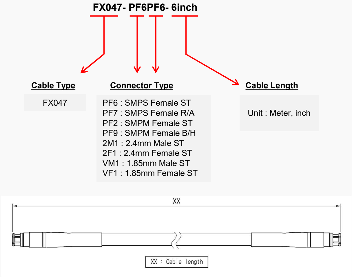
SMPS(F) S/T Connector(67 GHz)
